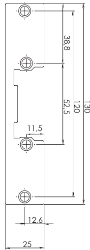
P (12)
