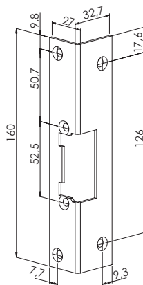
F53 (16)
