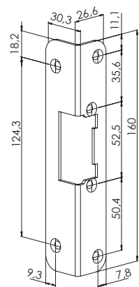
F54 (17)
