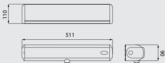
Universal arm
