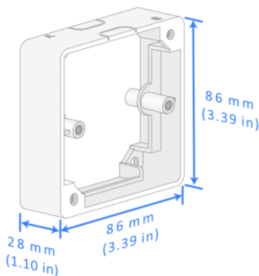
Figura 1-2 Dimensiones Recomendadas del Soporte
