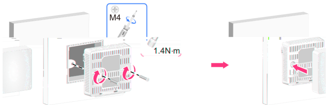
Gambar 1-4 Mengamankan Perangkat ke Kotak Sambungan
