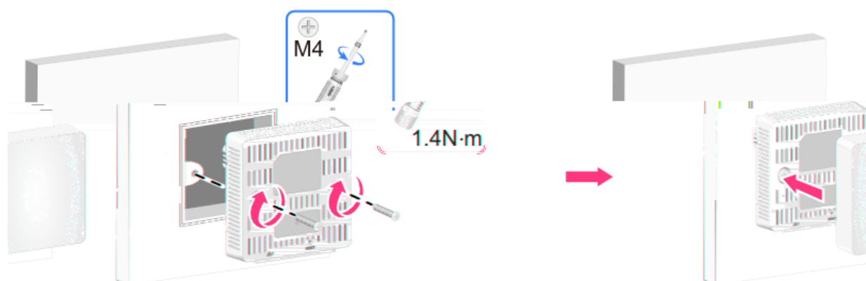
Figura 1-4 Fixação do dispositivo na caixa de junção
