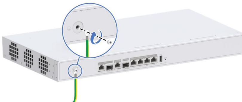
Figura 2-1 Conexão do cabo de aterramento
