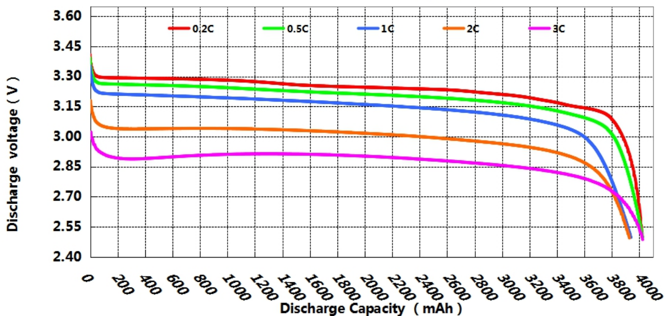
HDCF26650-4000mAh-3.2V (3C) 倍率温升图
