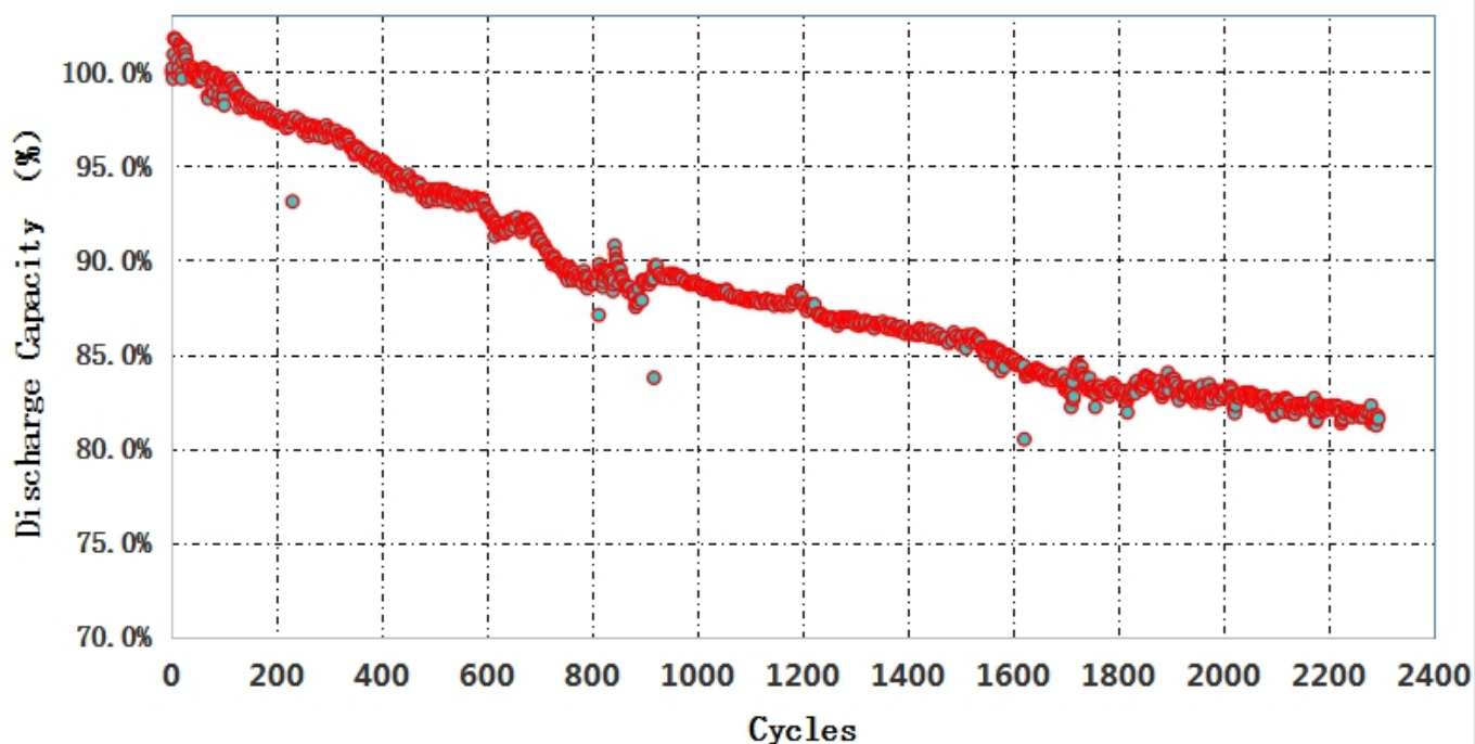
HDCF26650-4000mAh-3.2V (3C) 0.5C/1C循环曲线图
