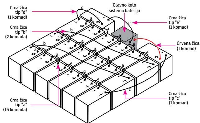
Dijagram povezivanja baterija
