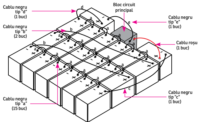
Diagrama de conectare a bateriilor
